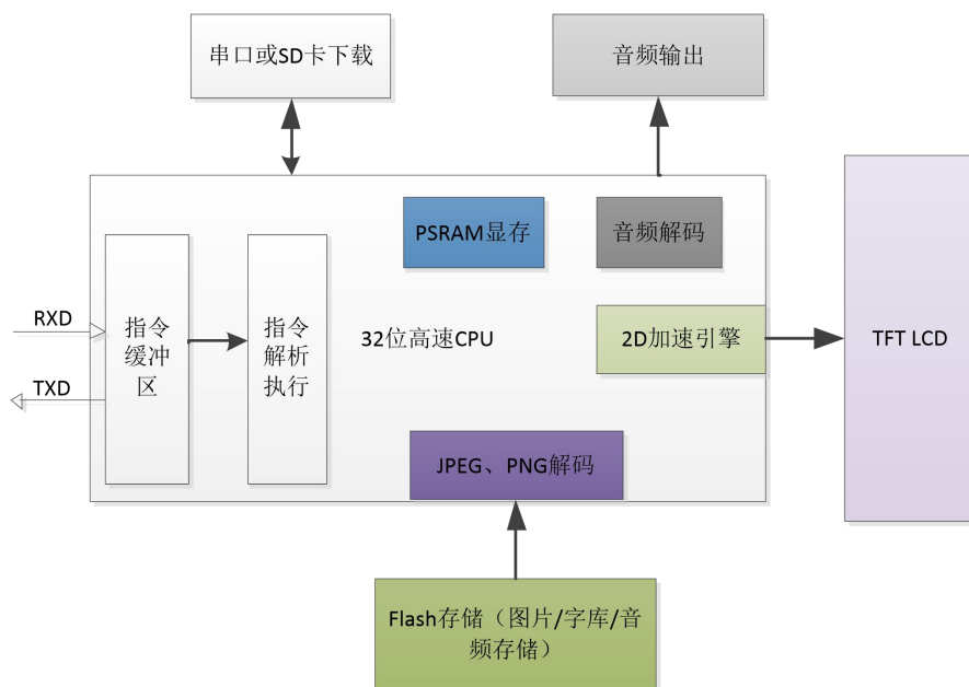
图 2-1 DB 系列串口屏内部结构图
