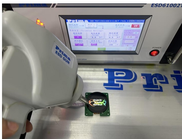
图 5-2 ESD 测试图
