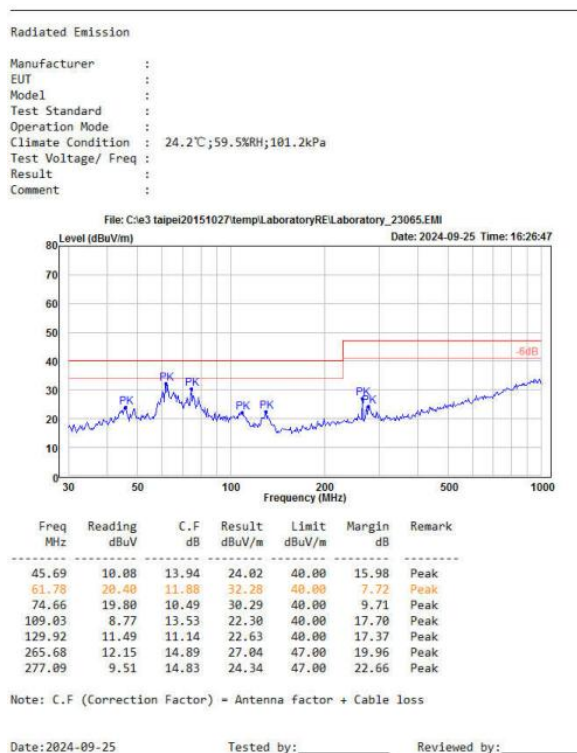
图 5-7 辐射测试垂直方向
