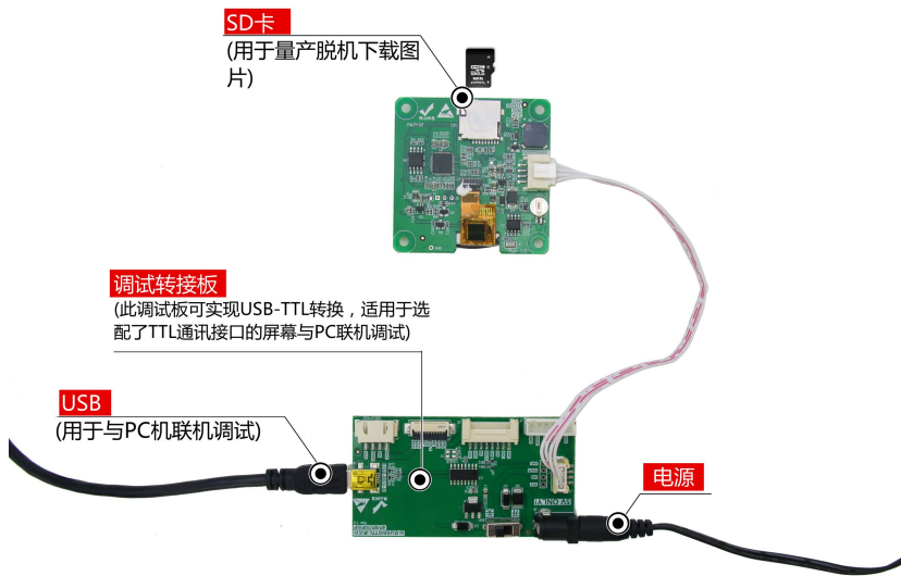
图 1-3 调试工具图
